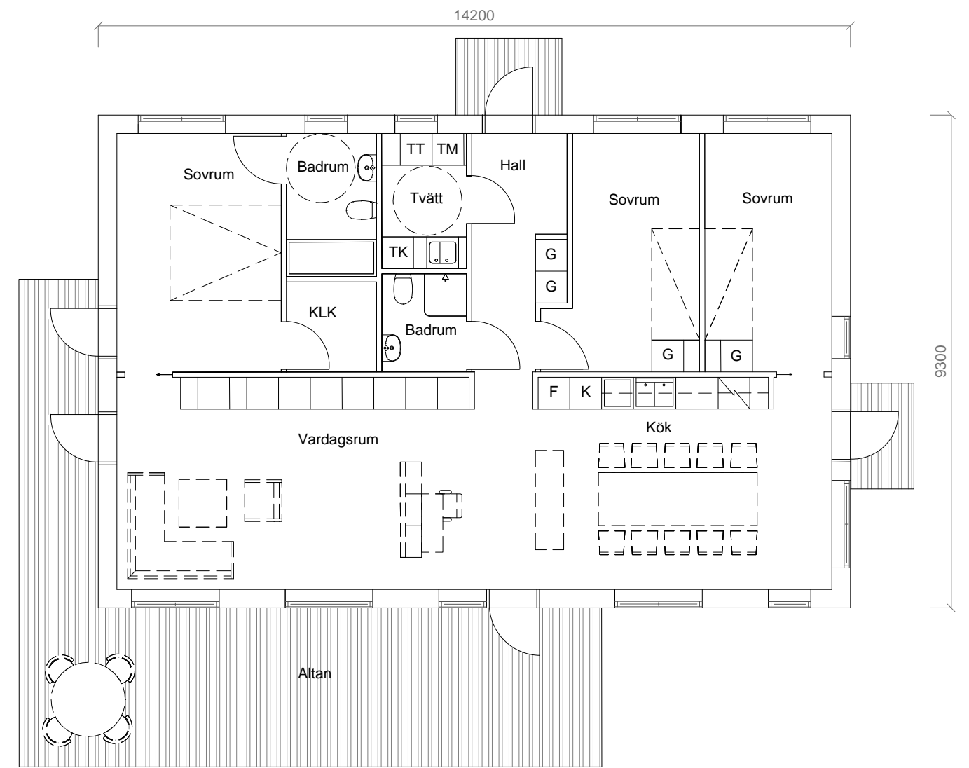
PLANRITNING
